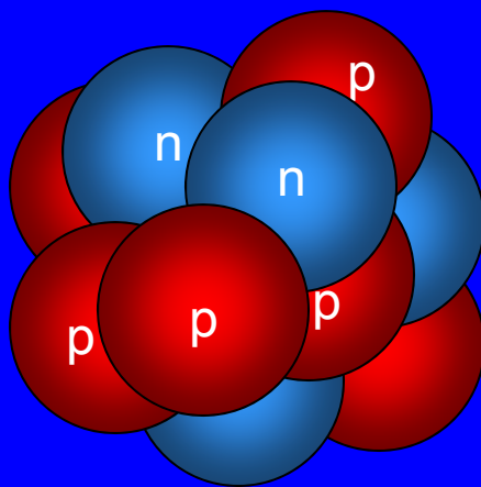
Parent Radionuclide
