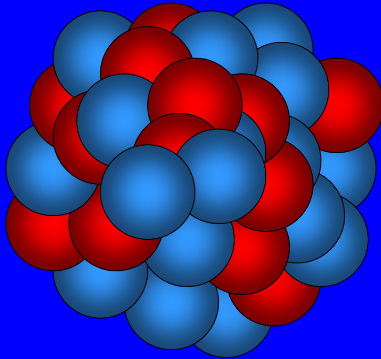
Parent Radionuclide
