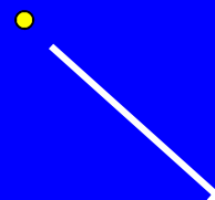
Neutrino
