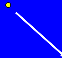
Neutrino
